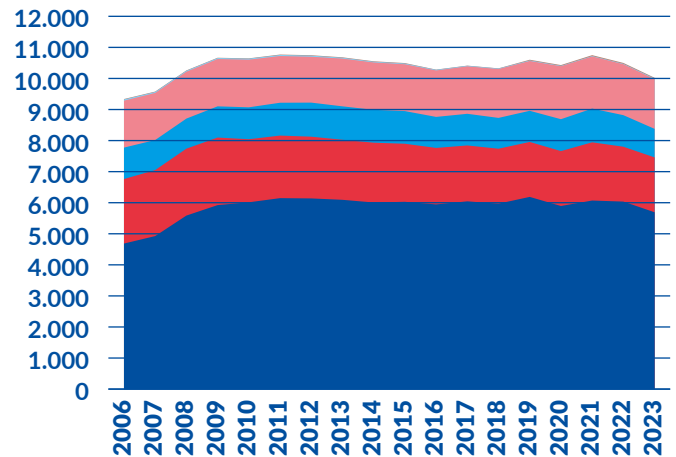
Ladekapazität von Trockengüterschiffen in den Rheinstaaen (in 1.000 Tonnen)
