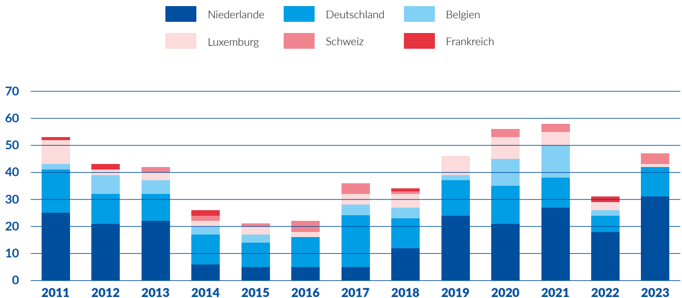
ABBILDUNG 10: NEUE TANKSCHIFFE AUF DEM MARKT PRO REGISTERLAND (ZAHLEN, 2011-2023)
