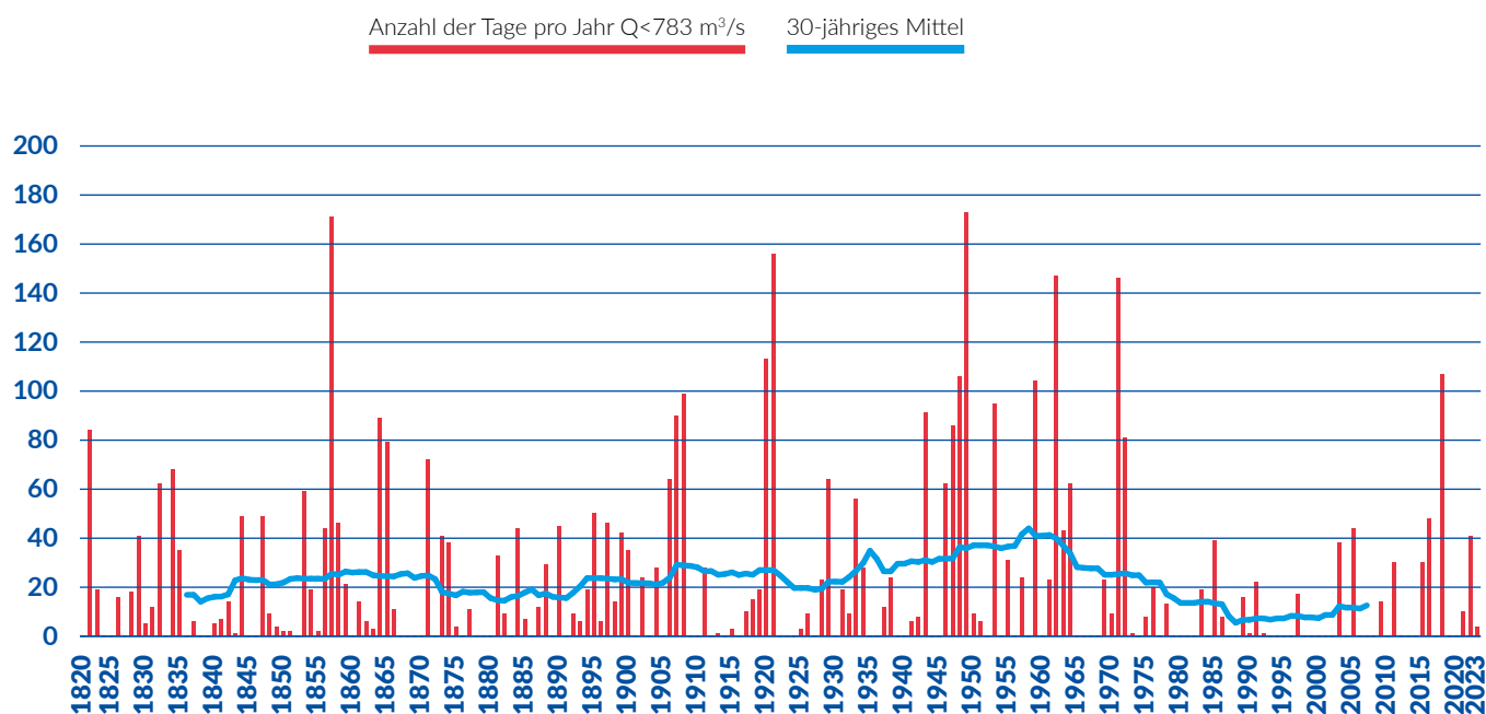
ABBILDUNG 3: ANZAHL DER TAGE PRO JAHR MIT EINEM ABFLUSS Q < 783 \text{ m}^3/\text{s} * BEI KAUB, MITTELREIN, EINSCHLIESSLICH 30-JÄHRIGES GLEITENDES MITTEL
